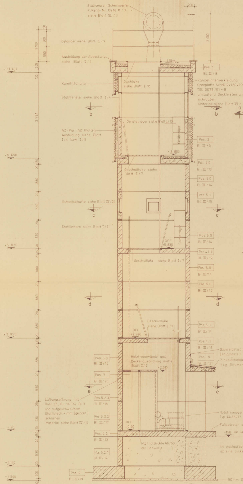
Schnitt a - a M 1:25
